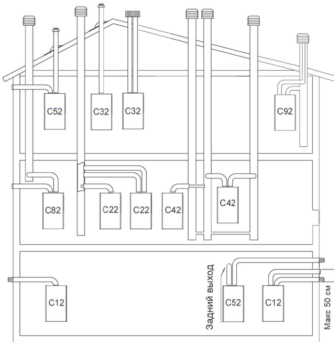
Рис.8 Дымоудаление типов С
